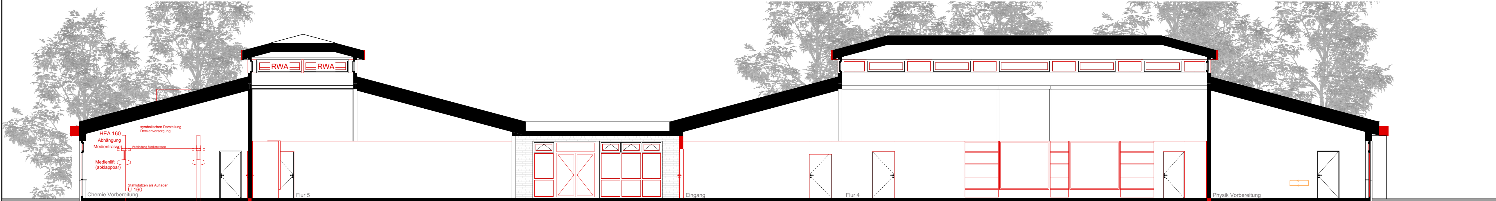
Schnitt 2-2
