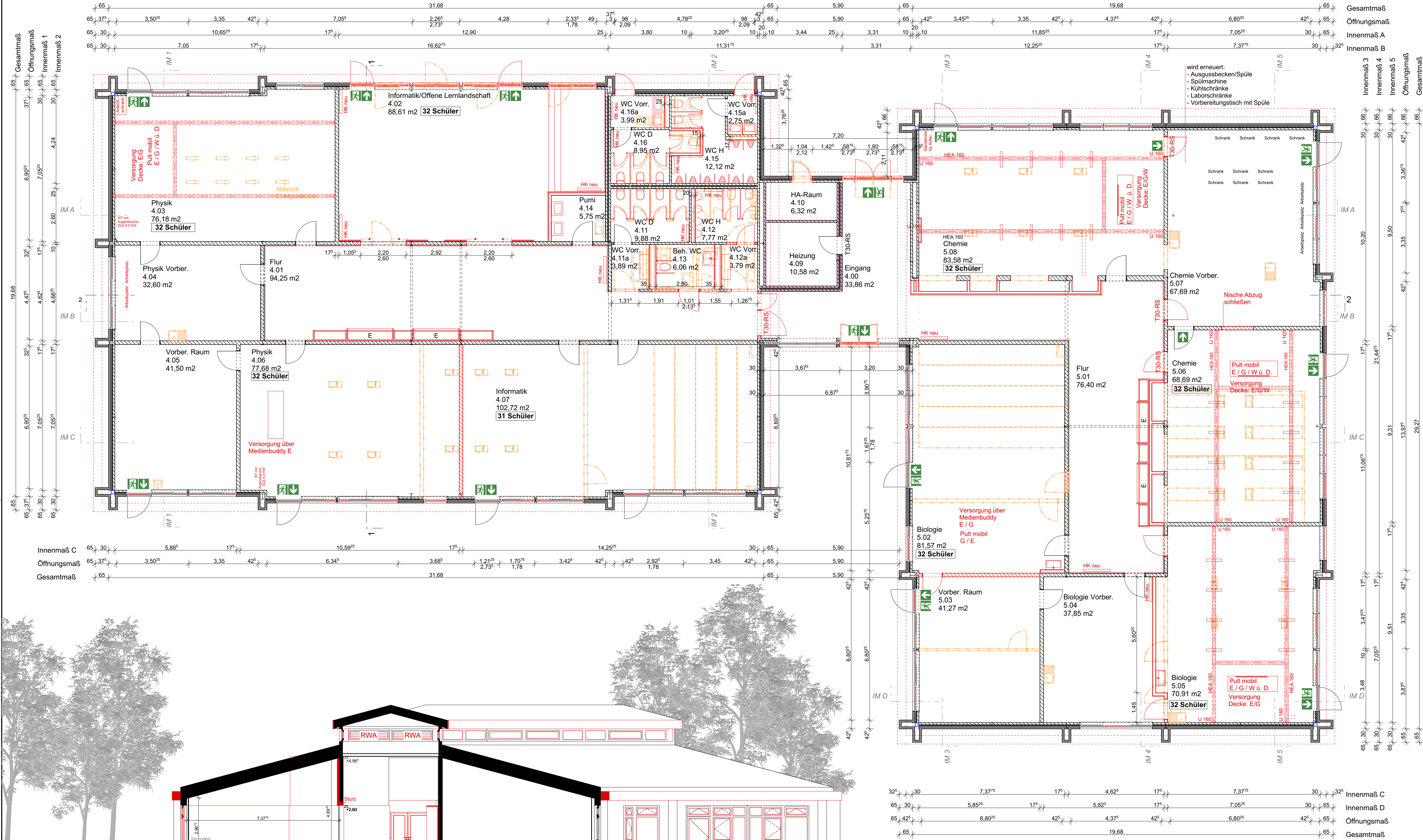
Schnitt 1-1
