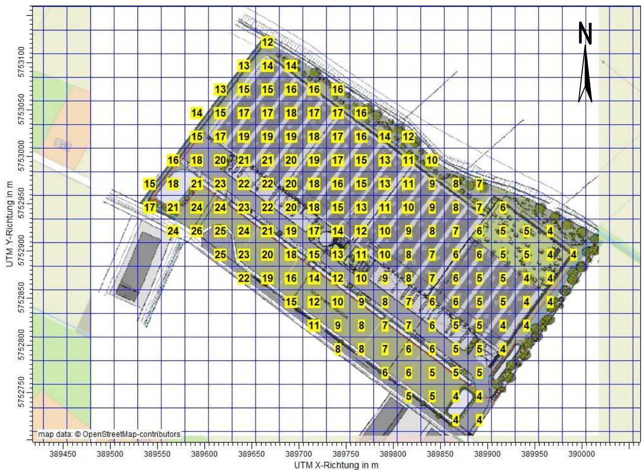
Abbildung 3: Gesamtbelastung IG_b durch die Betriebe TH 1 – TH 3 im genehmigten Bestand (inkl. Immissionsmindernder Maßnahme an einer Tierhaltungsanlage) in % der Jahresstunden, Seitenlänge: 25 m
