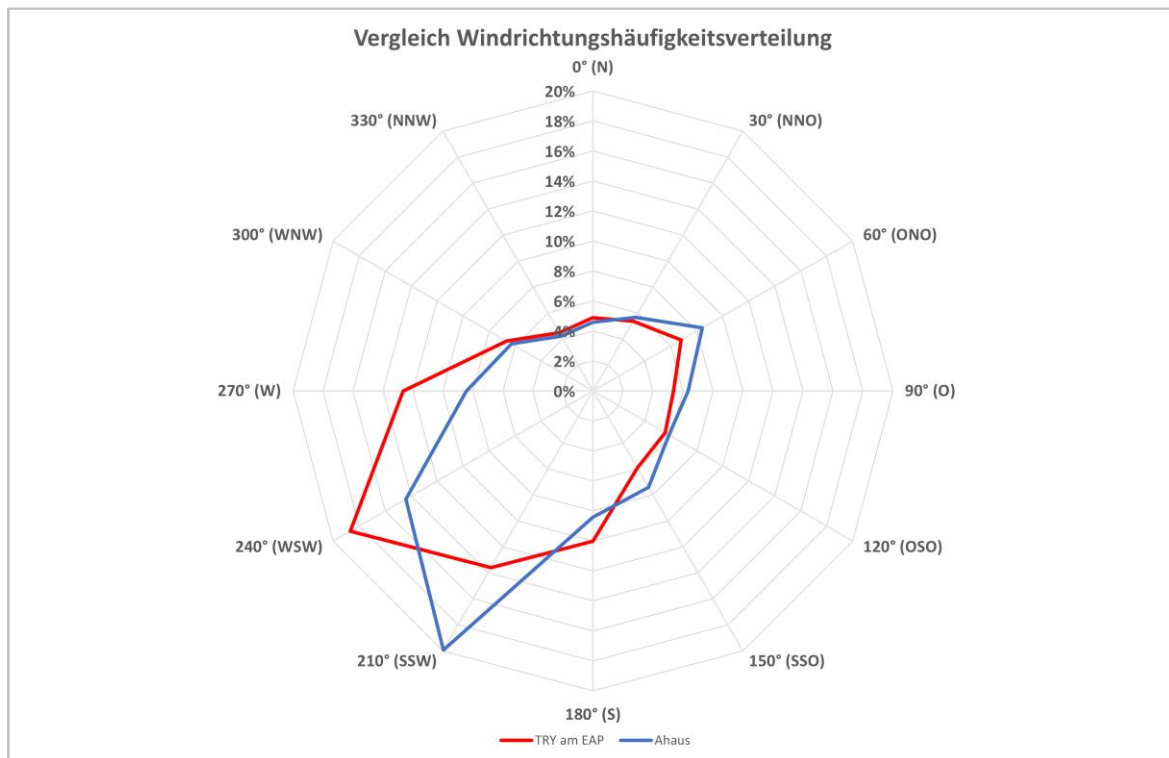
Abbildung 16: Vergleich Windrichtungsverteilung für EAP und Wetterstationen Ahaus
