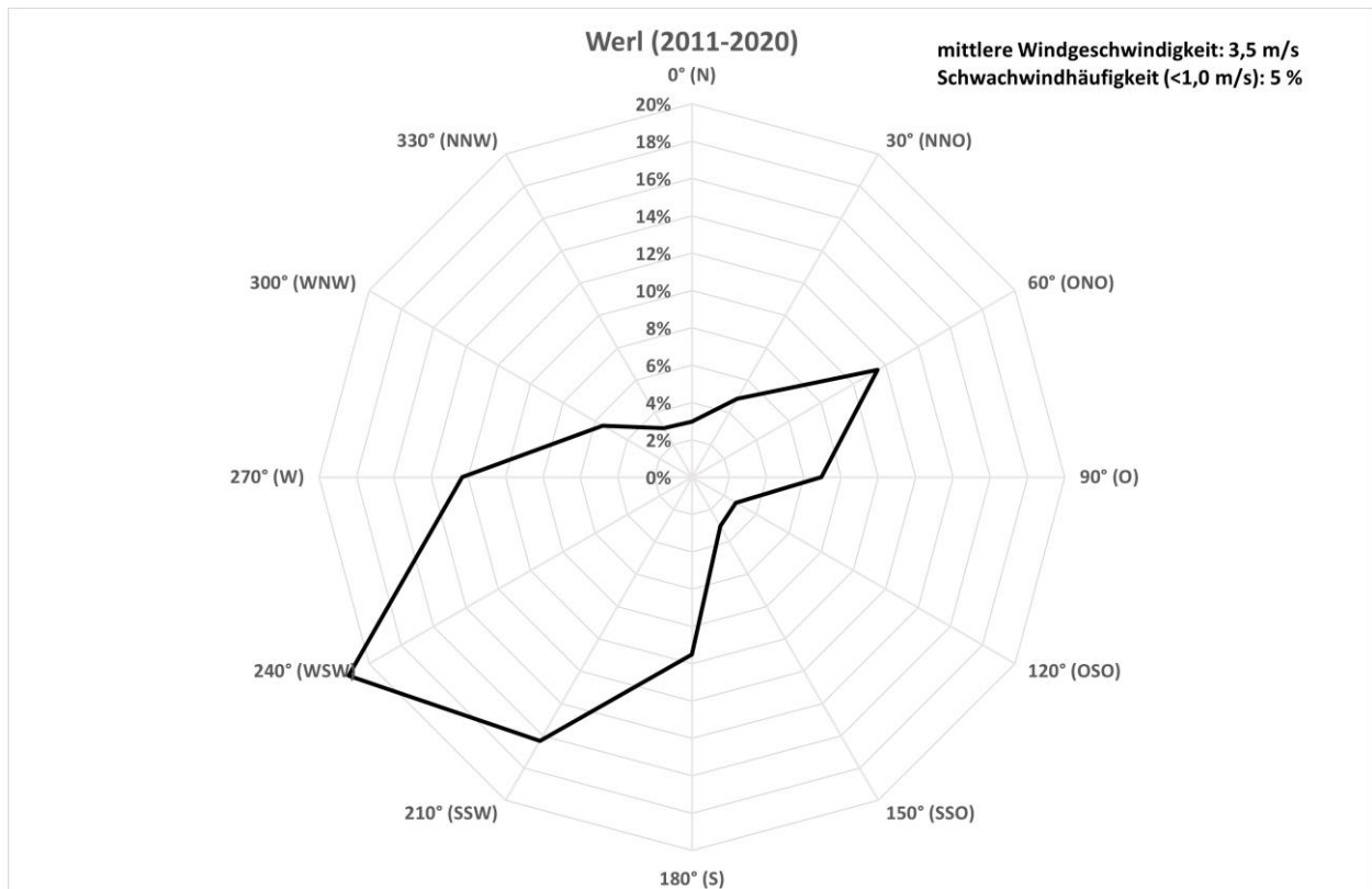
Abbildung 13: Windrichtungshäufigkeitsverteilung der Station Werl
