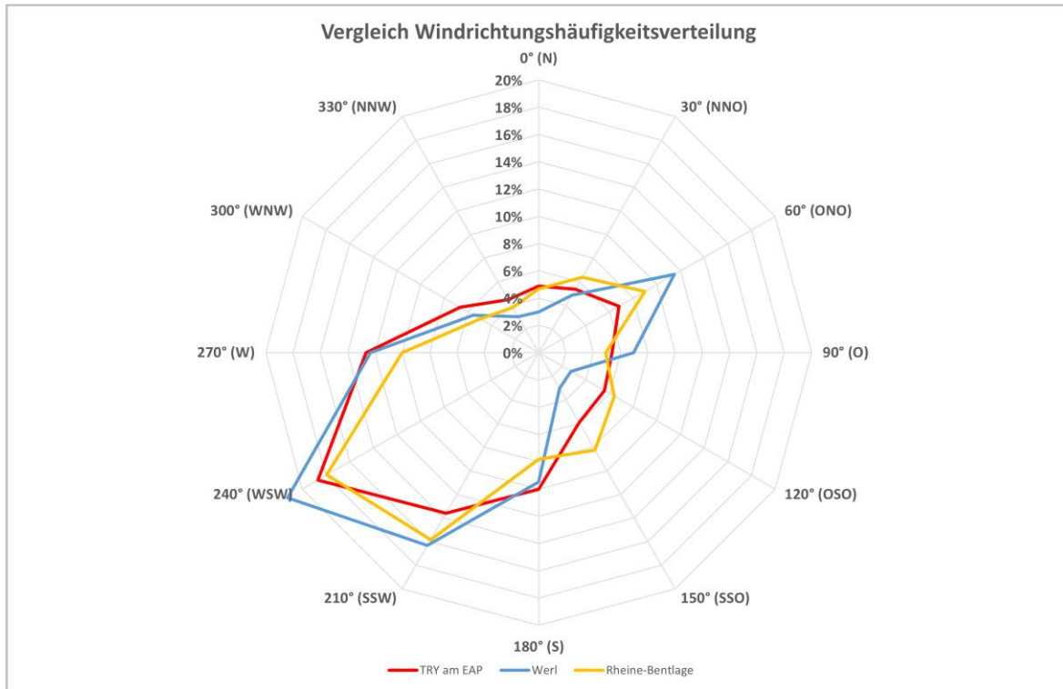
Abbildung 17: Vergleich Windrichtungsverteilung für EAP und Wetterstationen Werl und Rheine-Bentlage
