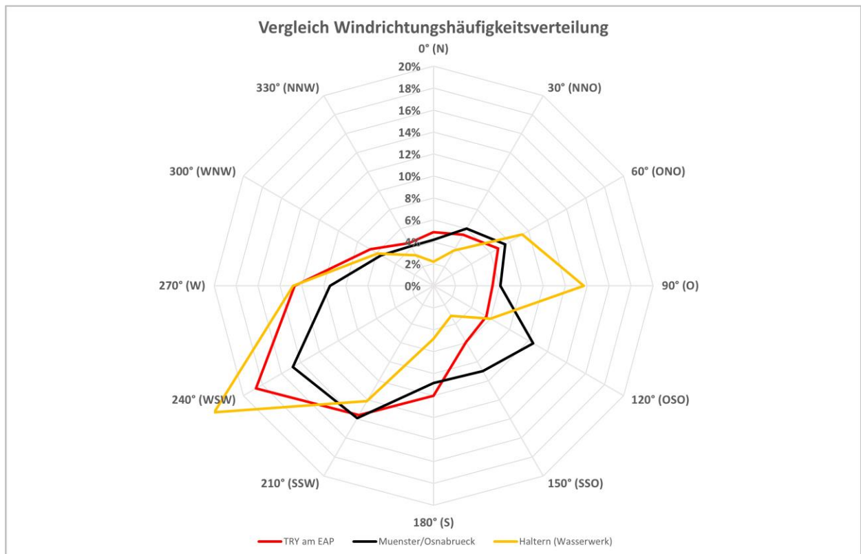
Abbildung 15: Vergleich Windrichtungsverteilung für EAP und Wetterstationen Münster/Osnabrück und Haltern (Wasserwerk)
