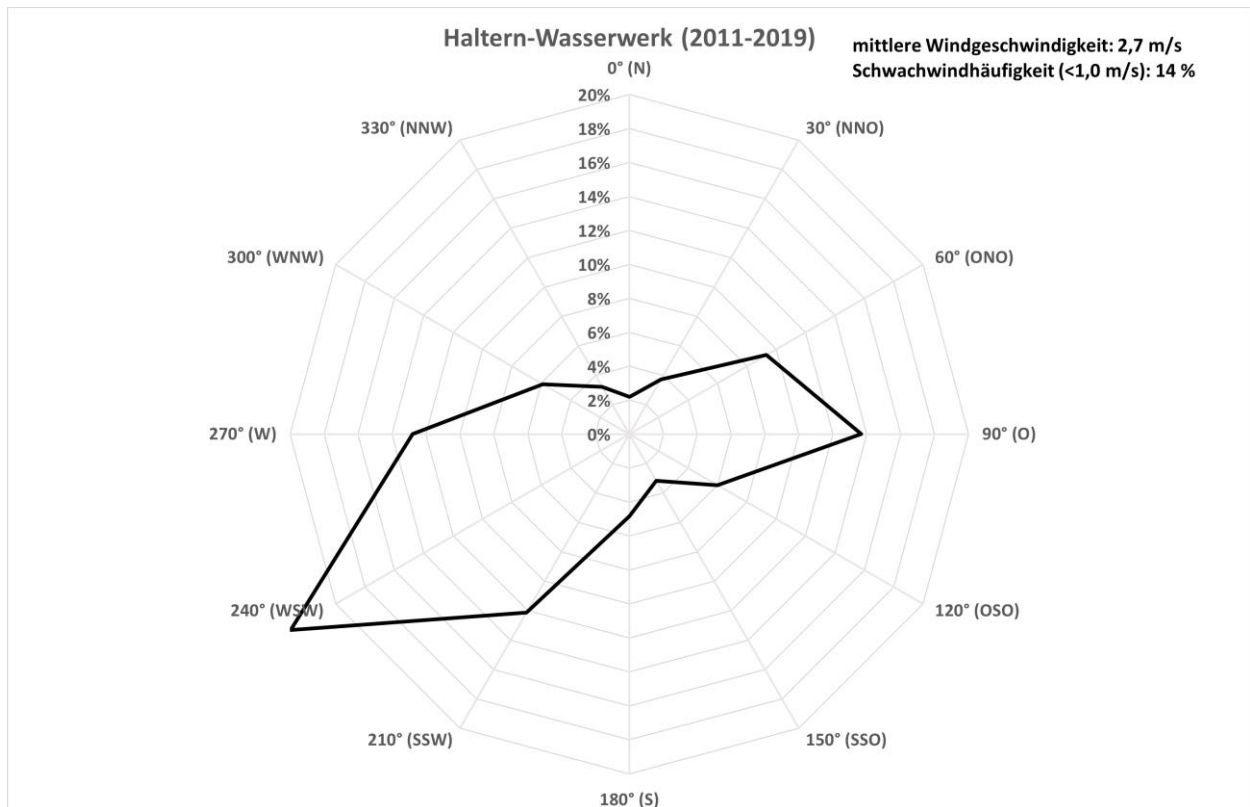
Abbildung 10: Windrichtungshäufigkeitsverteilung der Station Haltern (Wasserwerk)
