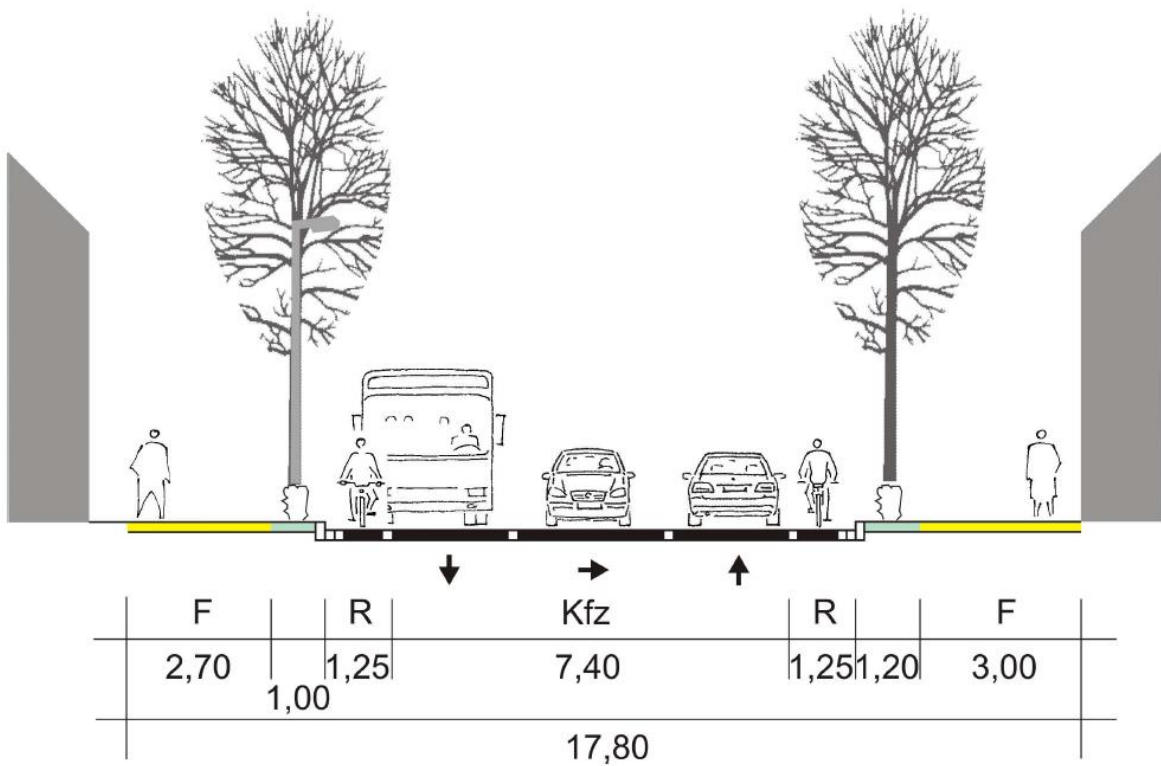
Abb. 51 Querschnittvariante 1: Markierung von Schutzstreifen
