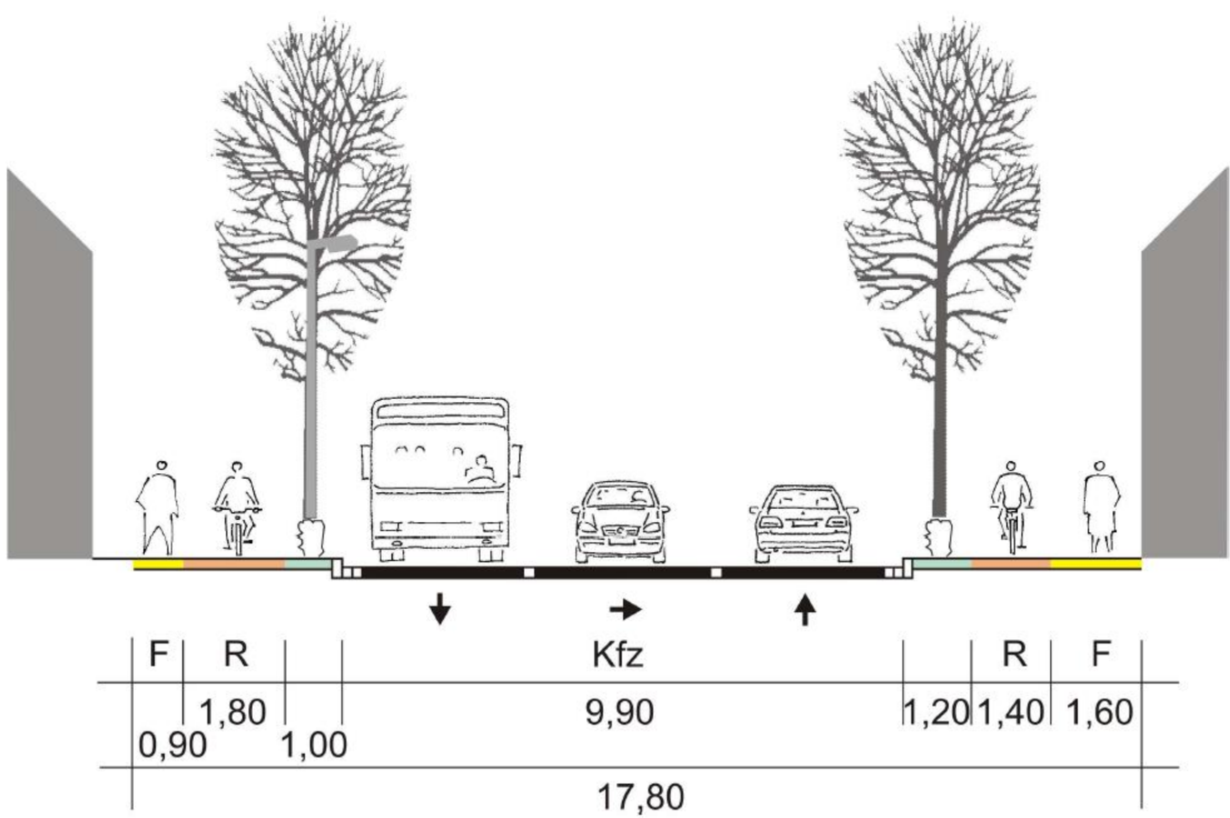
Abb. 50 Bestandsquerschnitt Daruper Straße
