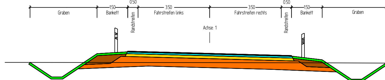
Querschnitt
