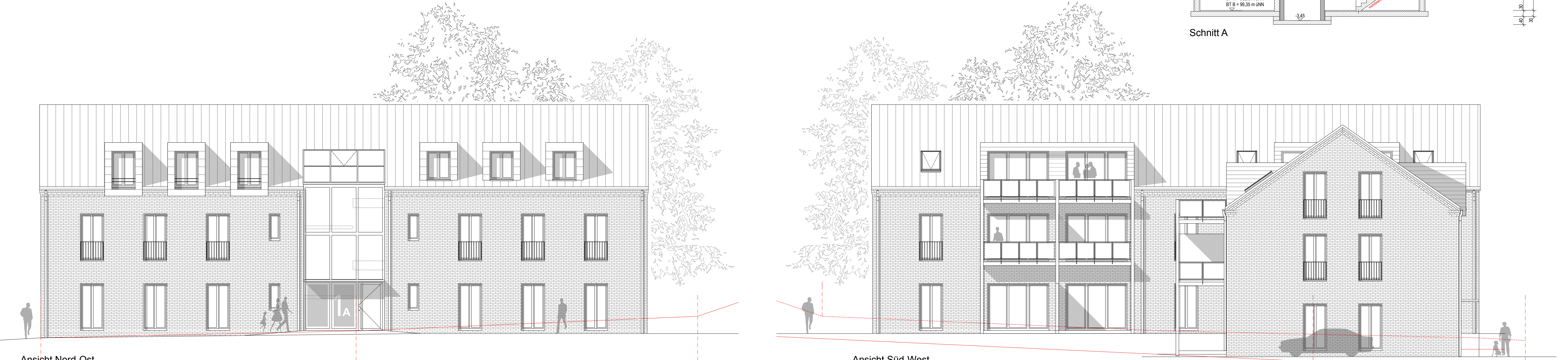
Ansicht Nord-Ost
