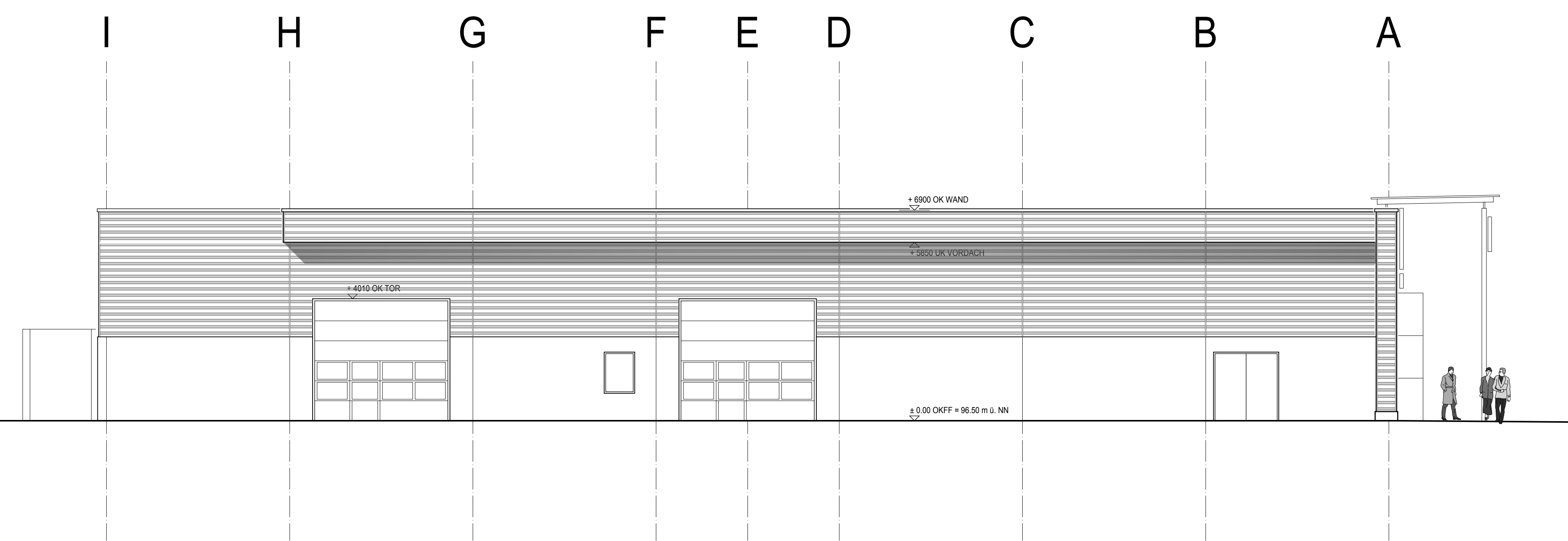
NORD - WEST ANSICHT
