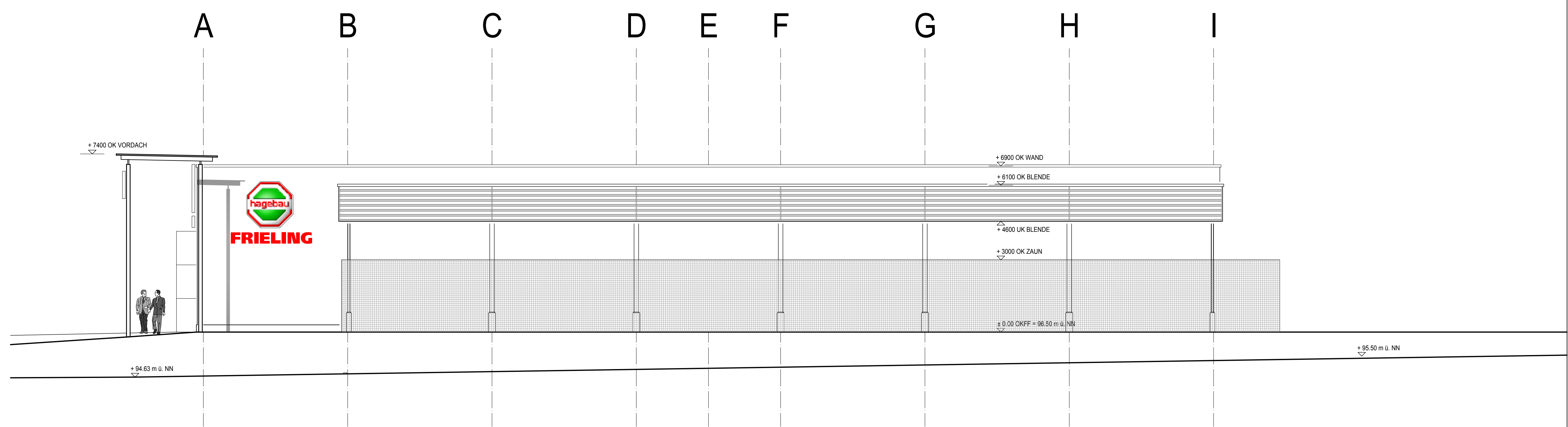
SÜD - OST ANSICHT
