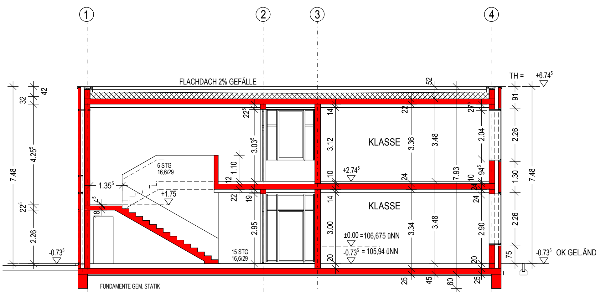
SCHNITT C - C
