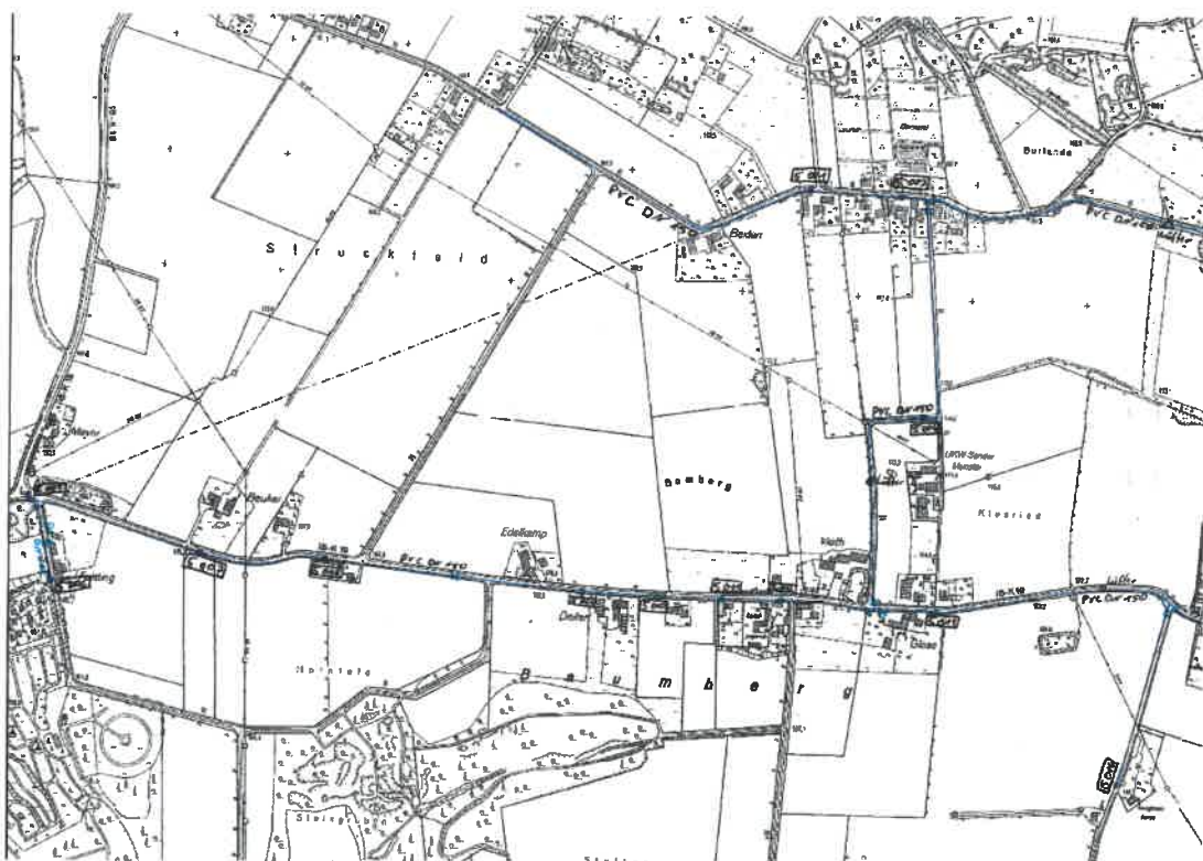
Abb. 13: Trinkwasserversorgungsnetz mit Hydranten, Detailplan Baumberg
