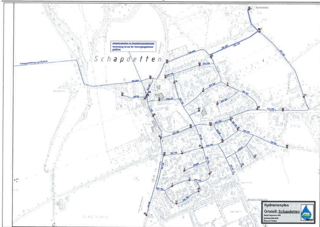
Abb. 12: Trinkwasserversorgungsnetz mit Hydranten, Detailplan Schapdetten
