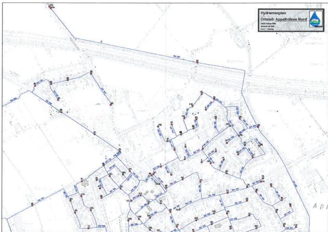
Abb. 10a: Trinkwasserversorgungsnetz mit Hydranten, Detailplan Appelhüsen Nord
