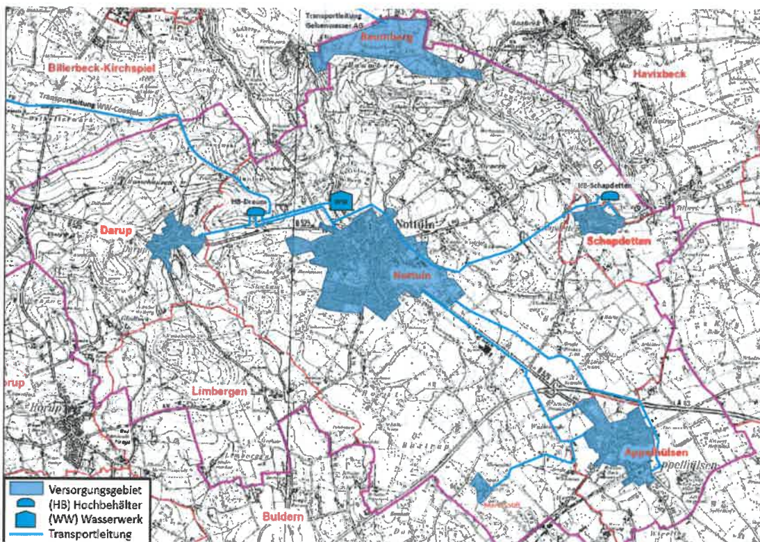
Abb. 7: Trinkwasserversorgungsnetz; Transportleitungen und Teilgebiete, Übersicht
