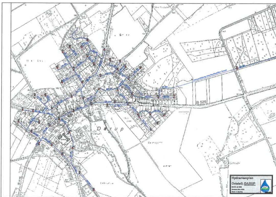
Abb. 11: Trinkwasserversorgungsnetz mit Hydranten, Detailplan Darup
