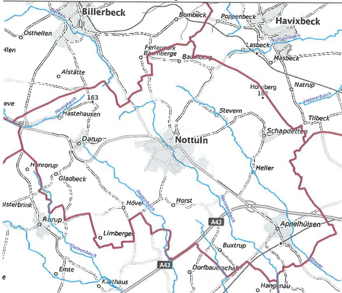
Abb. 1: Gemeindegrenzen Nottuln ( www.elwasweb.nrw.de/elwas-web/index.jsf# vom 18.05.2018)
