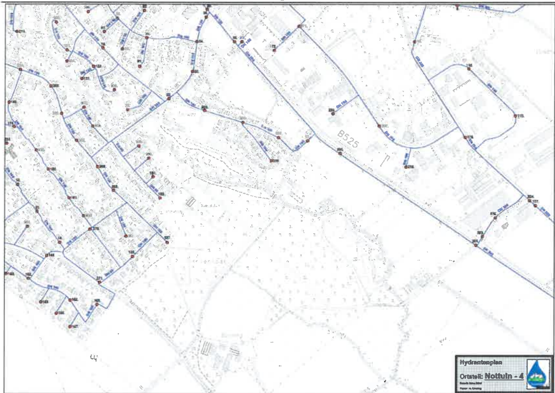
Abb. 9d: Trinkwasserversorgungsnetz mit Hydranten, Detailplan Nottuln Südost
