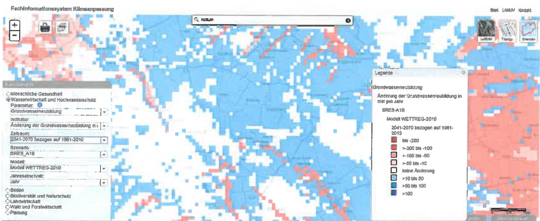
Abb. 19: Veränderung der Grundwasserneubildung Nottuln 2041-2070 / 1981-2010
