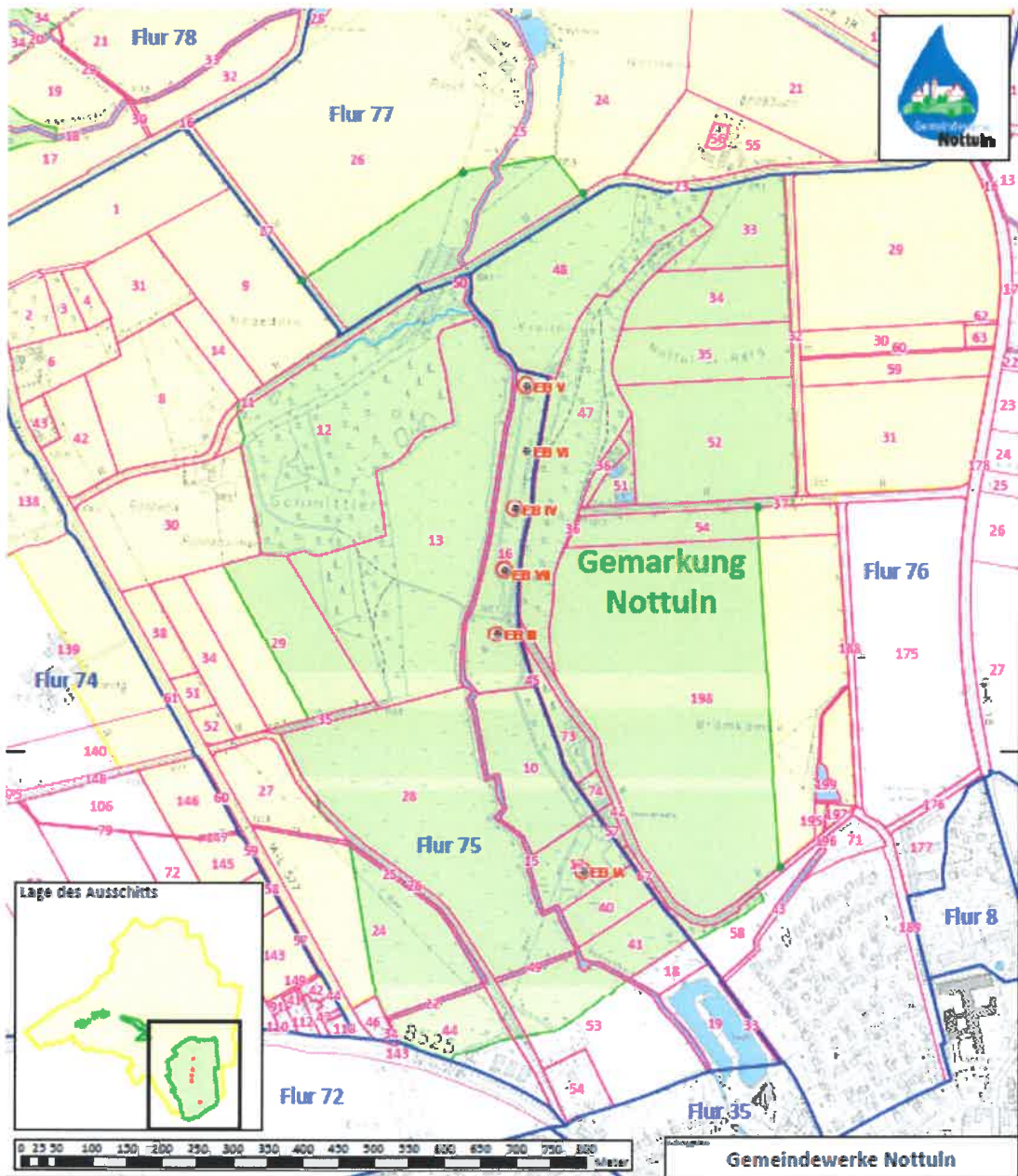
Abb. 5: Lageplan Entnahmehrinnen/Gewinnungsanlagen, Wasserwerk Nottuln
