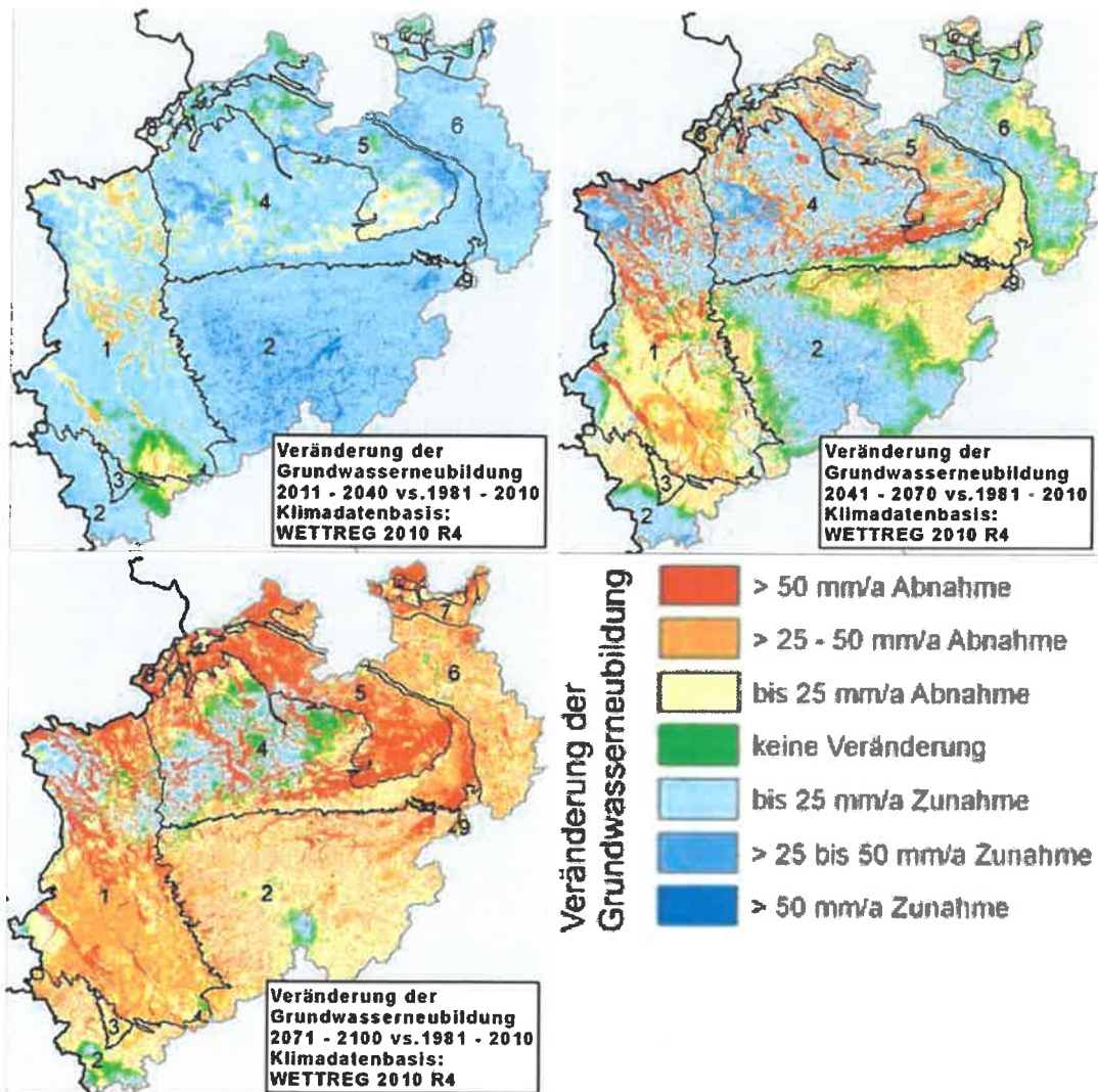
Abb. 17: Veränderung der Grundwasserneubildung in NRW, Übersicht
