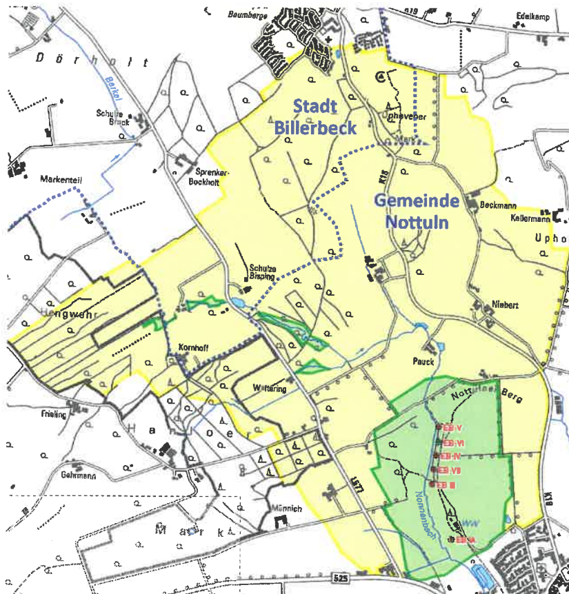
Abb. 4: Wasserschutzgebiet Nottuln
