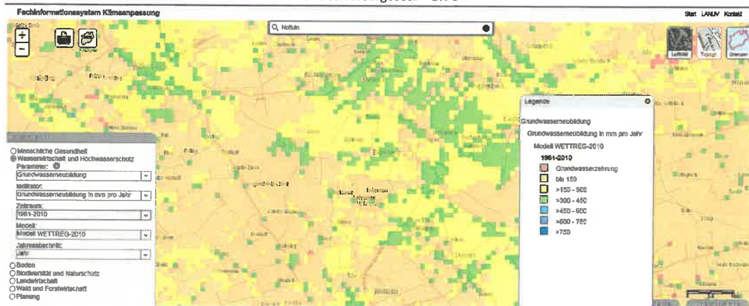
Abb. 16: Grundwasserneubildung 1981-2010 Nottuln
