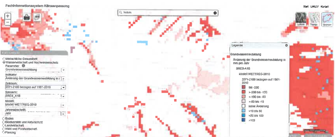
Abb. 20: Veränderung der Grundwasserneubildung Nottuln 2071-2100 / 1981-2010
