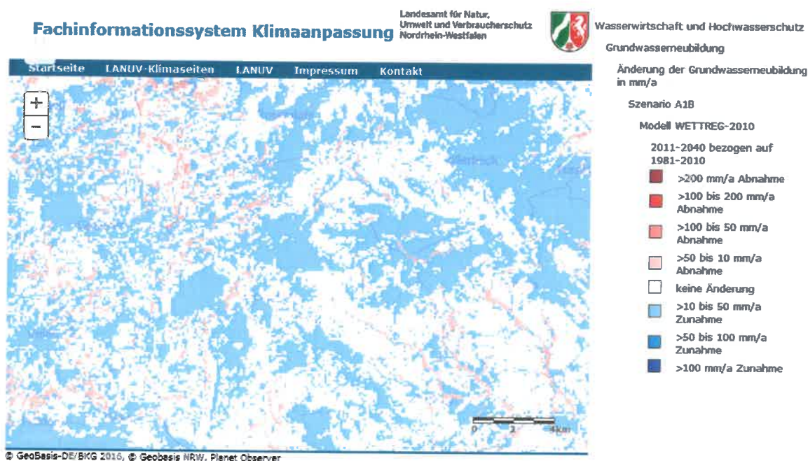
Abb. 22: Änderung der Grundwasserneubildung infolge des Klimawandels ( http://www.klimaanpassung-karte.nrw.de/ )
