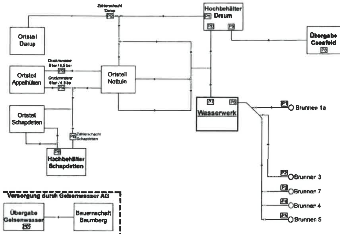
Abb. 8: Netzplan Nottuln, standardisiert
