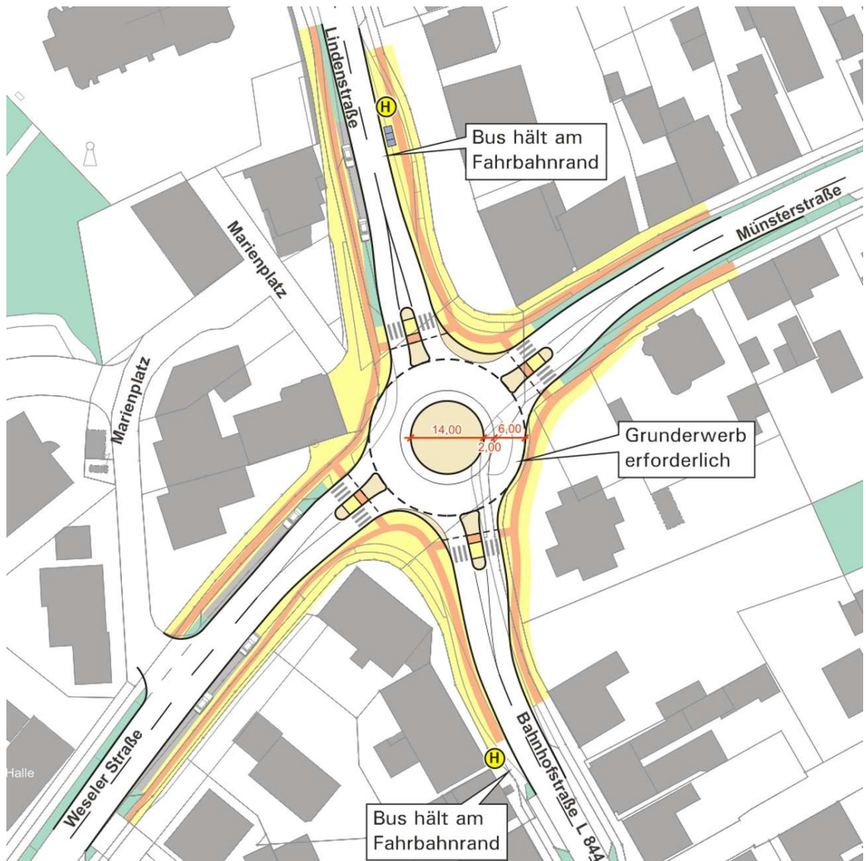
Abb. 68 Knotenpunktumgestaltung Variante 1: Kleiner Kreisverkehr (d = 30 m)
