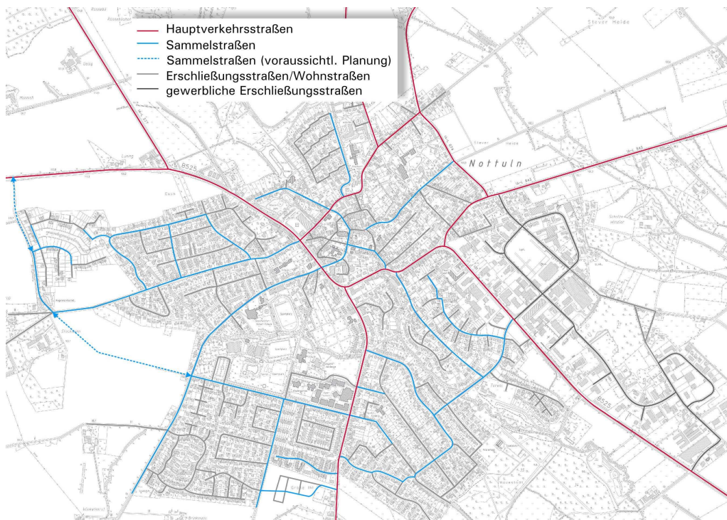
Abb. 13 Funktionale Gliederung des Straßennetzes für den Ortsteil Nottuln
