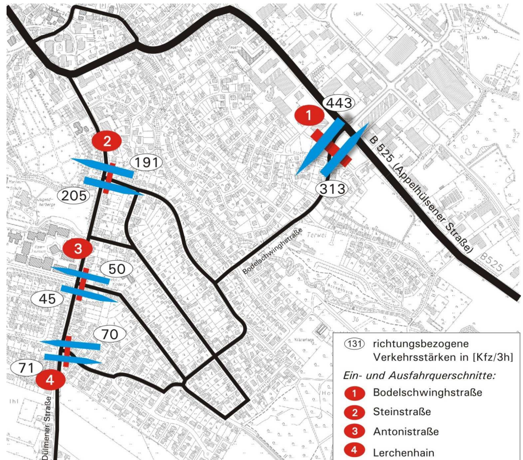
Abb. 18 Quell- und Zielverkehr für das Wohnquartier zwischen der B 525 und der Dülmener Straße
