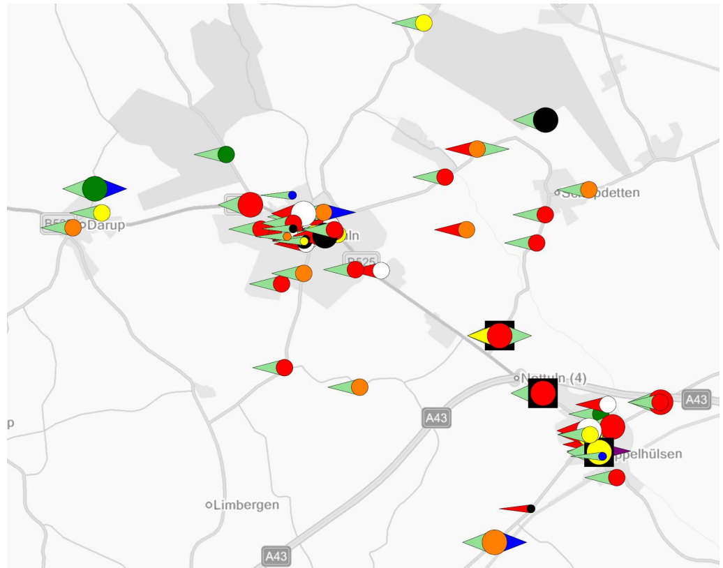
Abb. 26 Auszug aus der Unfalltypensteckkarte für die Gemeinde Nottuln
