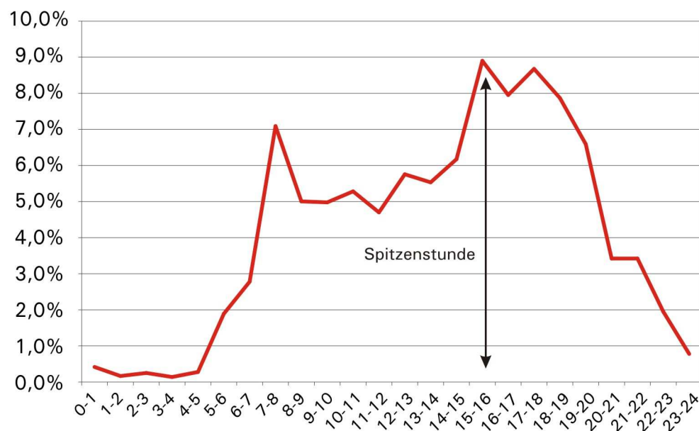
Abb. 3 Tagesganglinie für den Querschnitt Niederstockumer Weg
