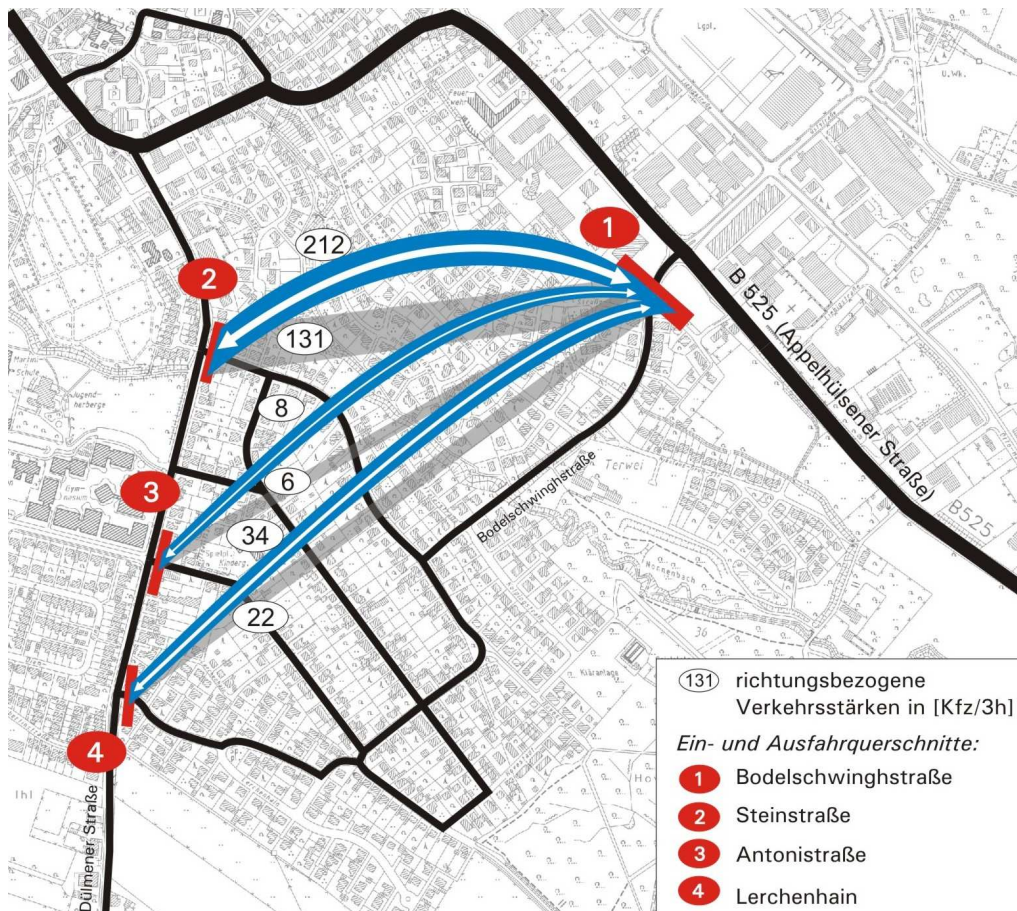
Abb. 17 Durchgangsverkehr im Wohnquartier zwischen der B 525 und der Dülmener Straße
