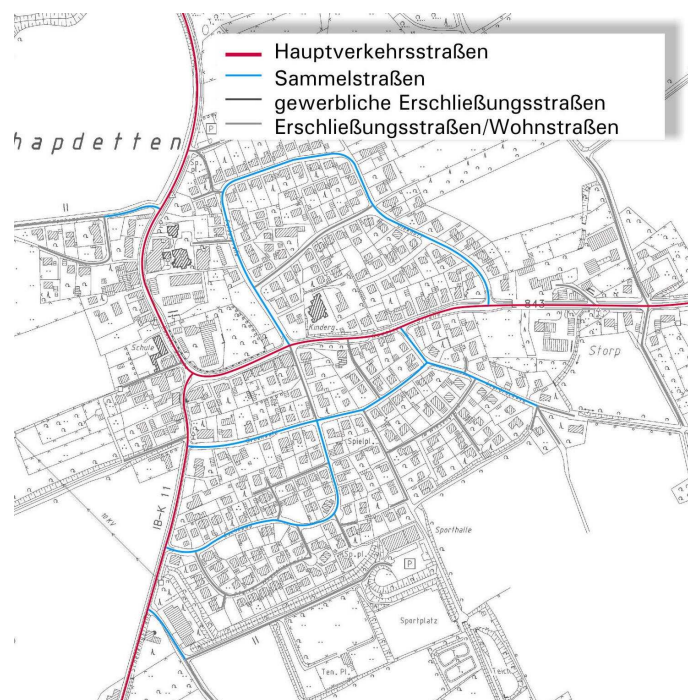
Abb. 16 Funktionale Gliederung des Straßennetzes für den Ortsteil Schapdetten
