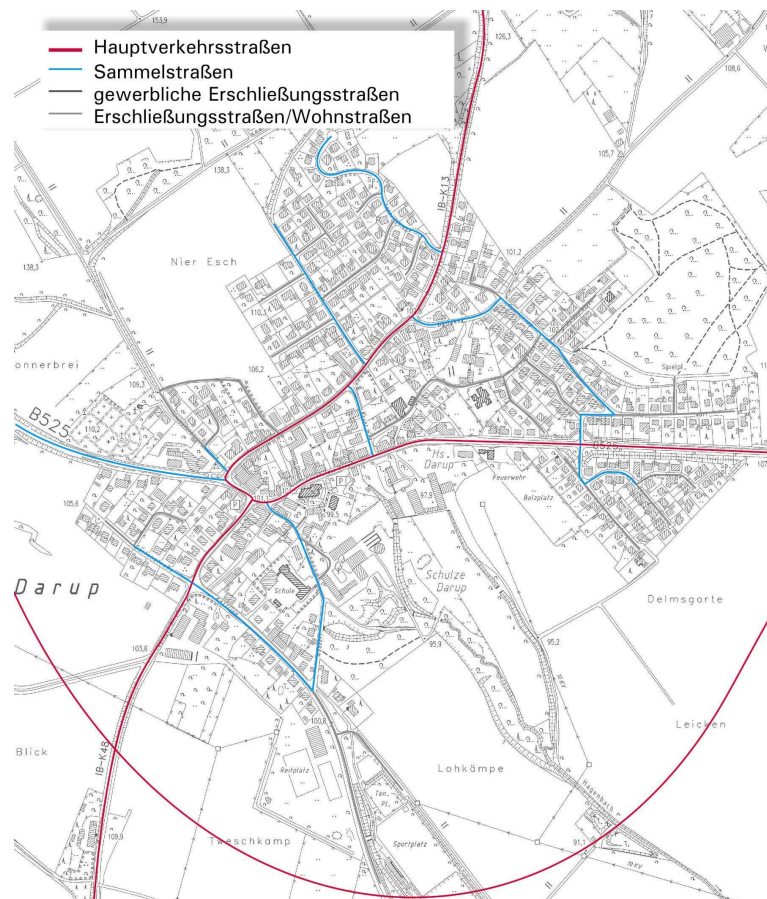
Abb. 15 Funktionale Gliederung des Straßennetzes für den Ortsteil Darup
