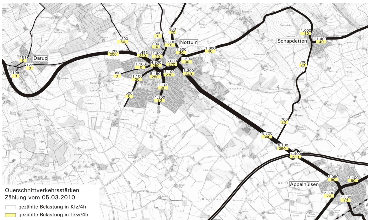
Abb. 4 Querschnittverkehrsstärken für den Zeitraum von 15:00 Uhr bis 19:00 Uhr in der Gemeinde Nottuln
